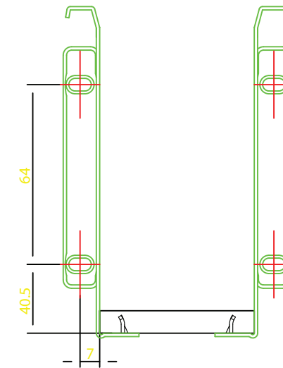
前连接件安装尺寸
